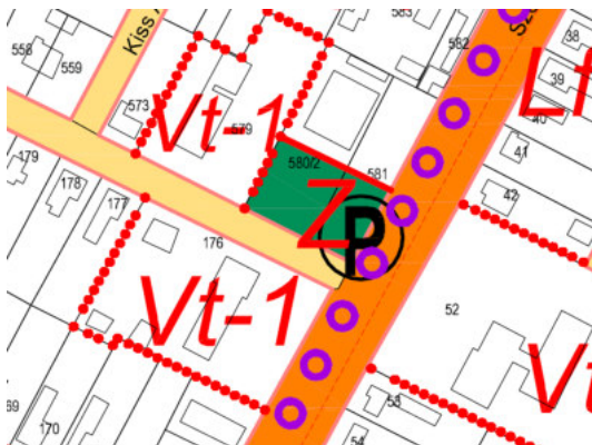
hatályos szabályozási terv részlete
